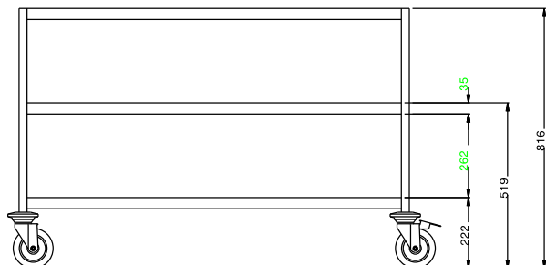
Zepředu
